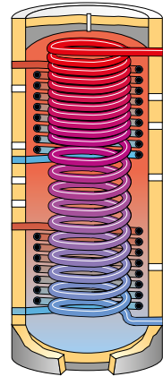
Hygienespeicher „Thermoplus“ lieferbar mit 500 l, 800 l und 1000 l Gesamtvolumen
